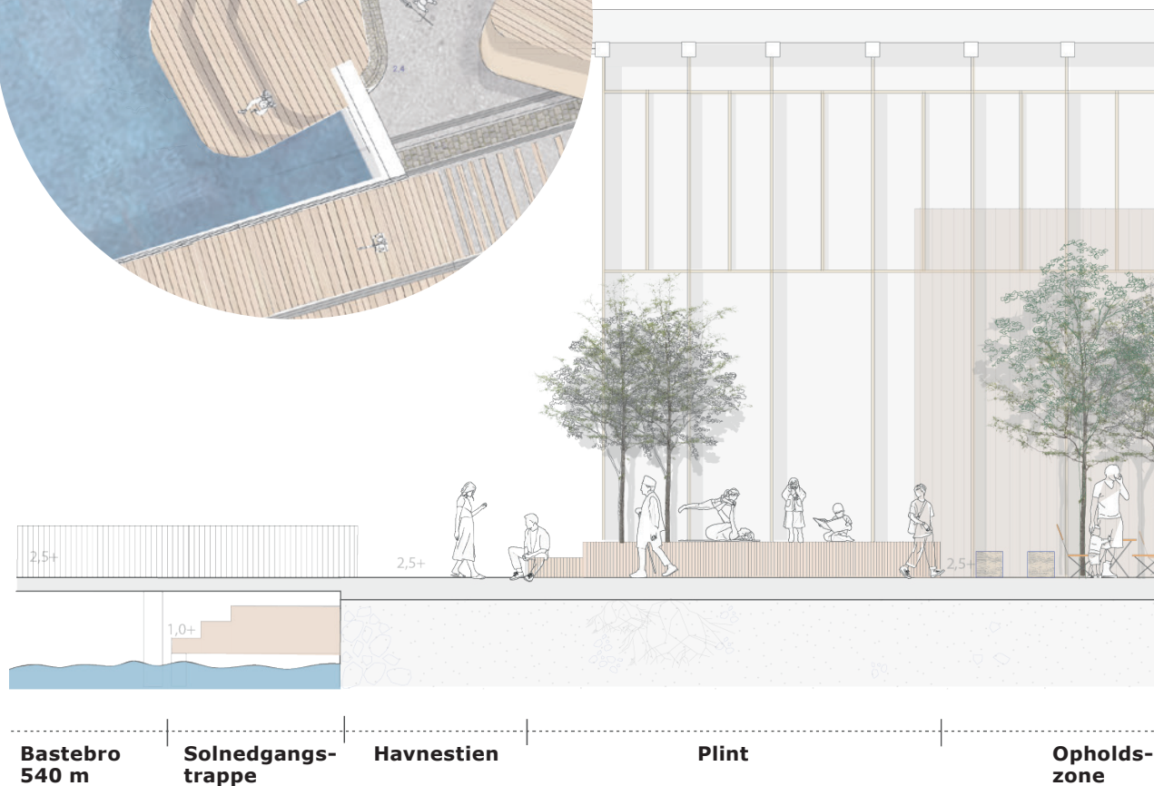
FIGUR 12. LÆNGDESNIET AF SOLNEDGANGS-TRAPPEN
